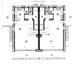
Ebene 0, M 1:400
