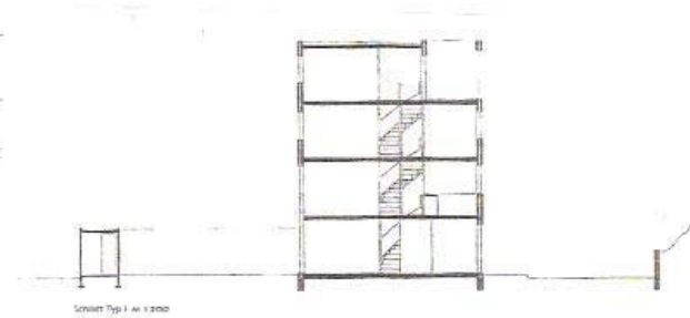
Schnitt Typ I M 1:200
