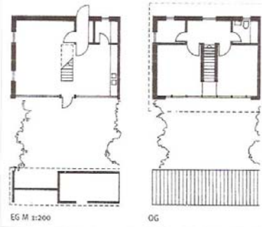
EG M 1:200
